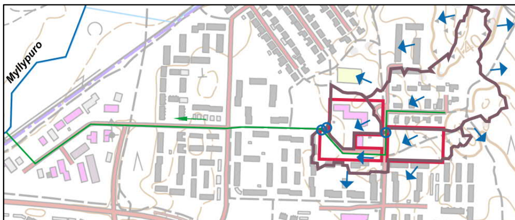
Kuva 2 Suunnittelualueen nykyiset valuma-alueet, valuma-alueiden purkupisteet, pintavalunnan suunta sekä päävirtausreittinä toimiva nykyinen hulevesiviemäri, joka purkaa Myllypuroon.
